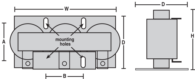
75-500 HP; 110-600 Amp
