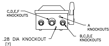
NEMA TYPE 1
