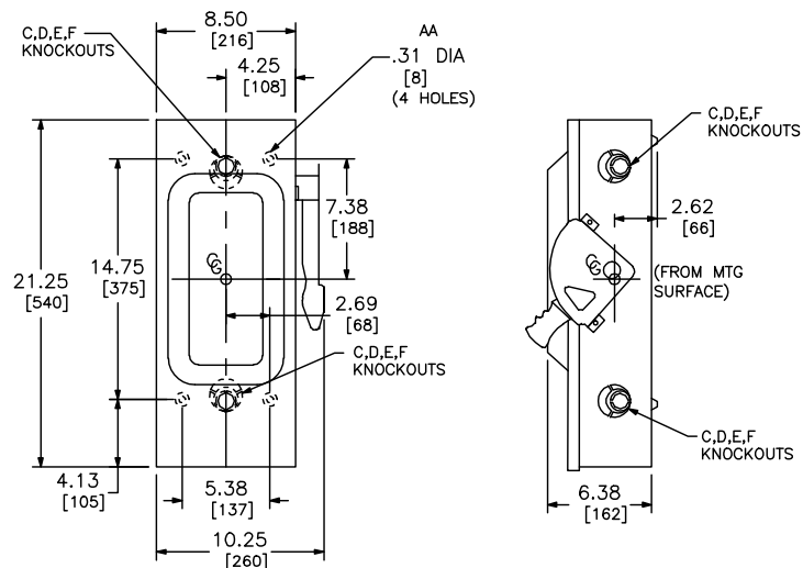
NEMA TYPE 1
